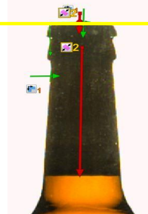
Unterfüllung schlecht
