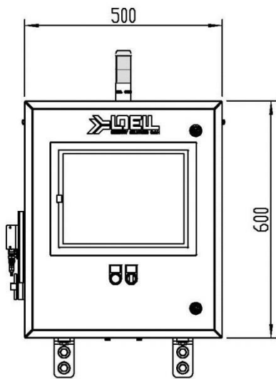
Vorderansicht
