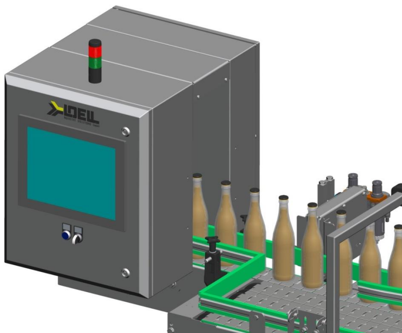
LIS - Füllhöhenkontrolle (Kamera)
